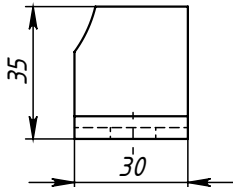
Поз.4 (Ушко)
