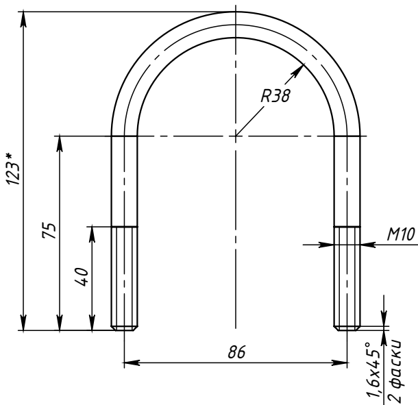
Поз.5 (Хомут)
