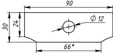
Поз.4 (Ушко) развертка
